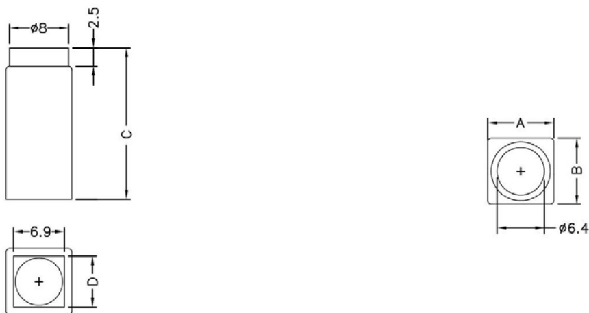
LSCD15 结构图
