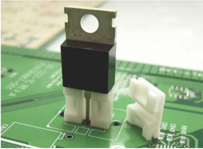
DTZ-35 结构图
