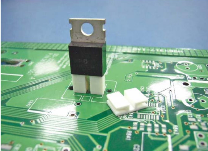
DTZ-8 结构图
