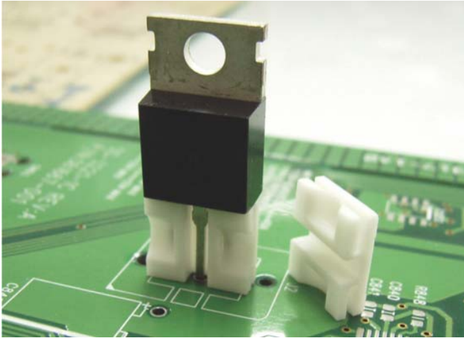
DTZ-38 结构图
