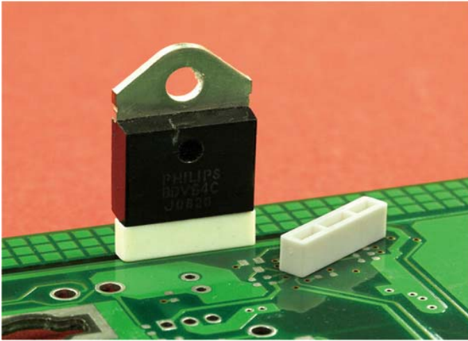
DTZ-68 结构图
