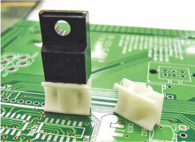
DTZ-44 结构图
