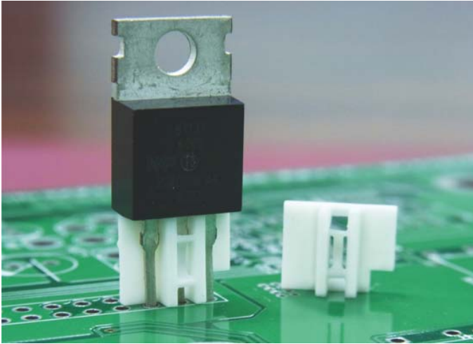
DTZ-21 结构图
