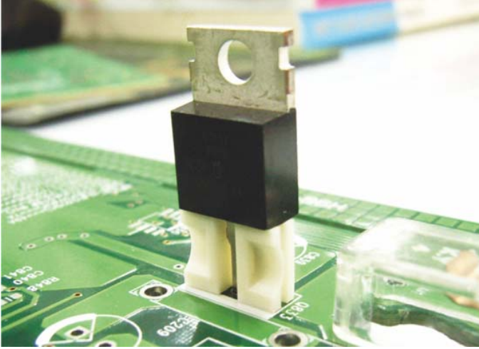
DTZ-13 结构图
