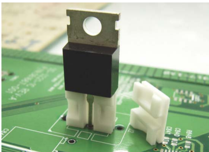
DTZ-33 结构图
