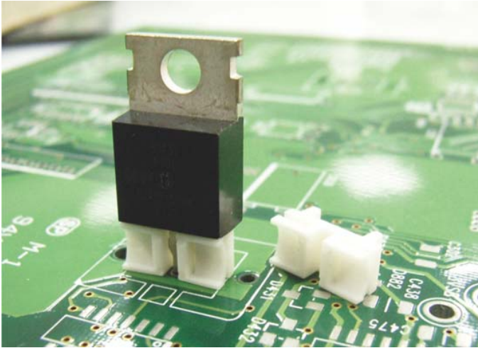
DTZ-19 结构图
