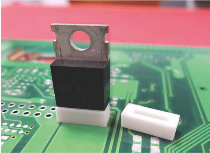
DTZ-54 结构图
