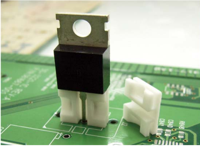
DTZ-71 结构图
