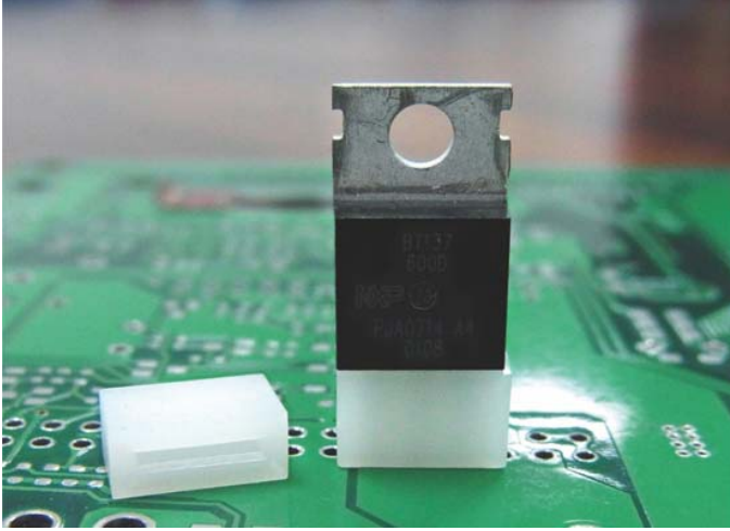
DTZ-4 结构图
