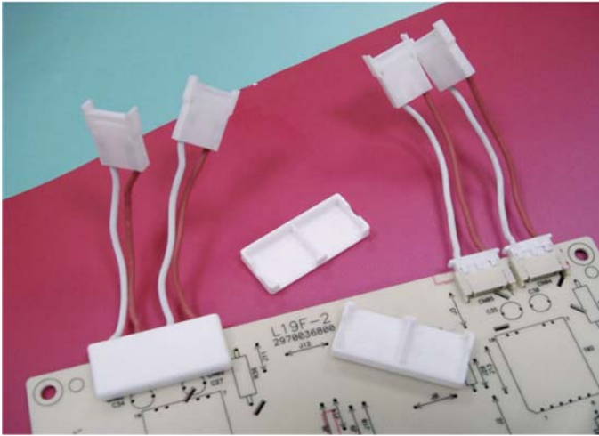
GFR-9 结构图
