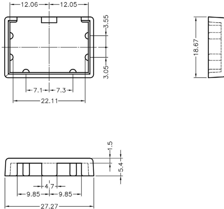
GFR-10 结构图
