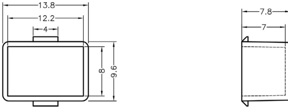
GFR-22 结构图
